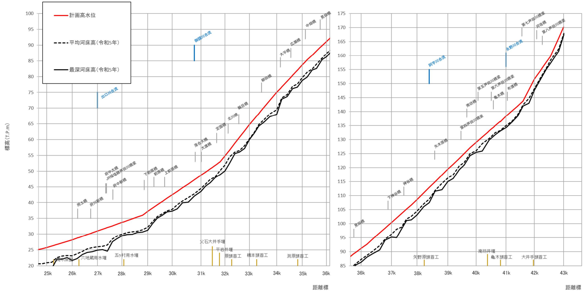
図 4-1 (2) 計画縦断図 (芦田川)
