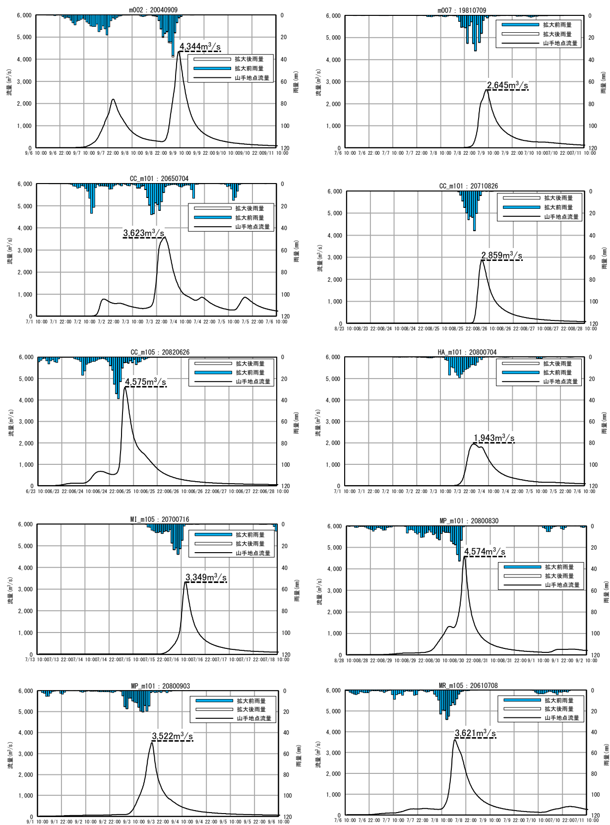
図 1-18 抽出したアンサンブル予測降雨波形のヒドログラフ（基準地点山手）
