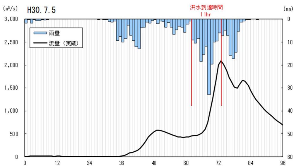
図 1-8(4) Kinematic Wave 法による洪水到達時間の検討
