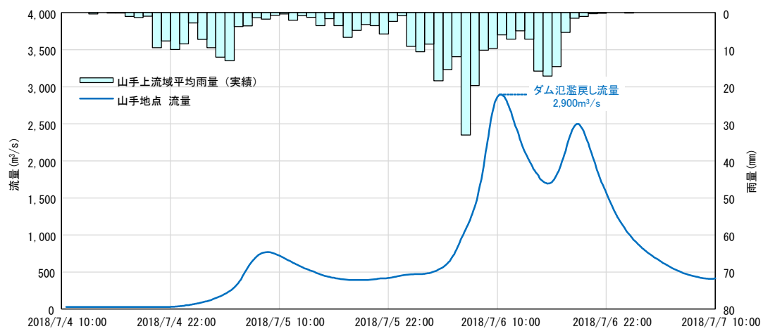
図 1-21 平成 30 年 7 月洪水（ダム氾濫戻し）の流量ハイドログラフ
