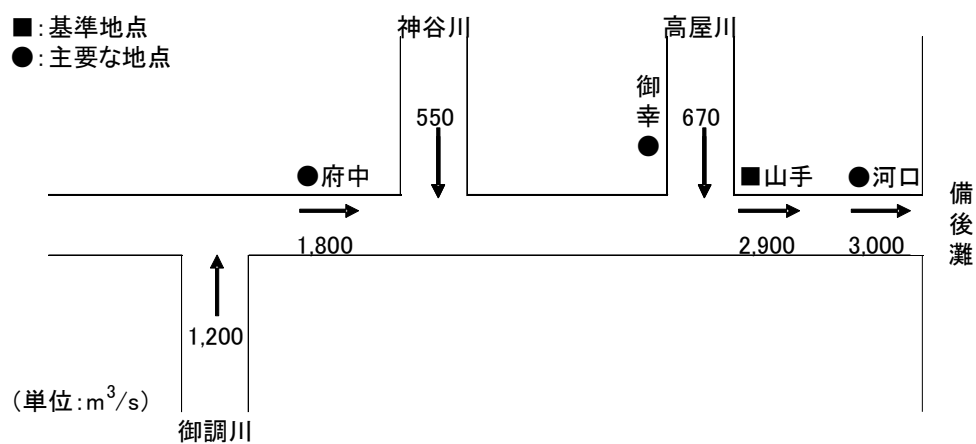
図 3-1 芦田川計画高水流量配分図
