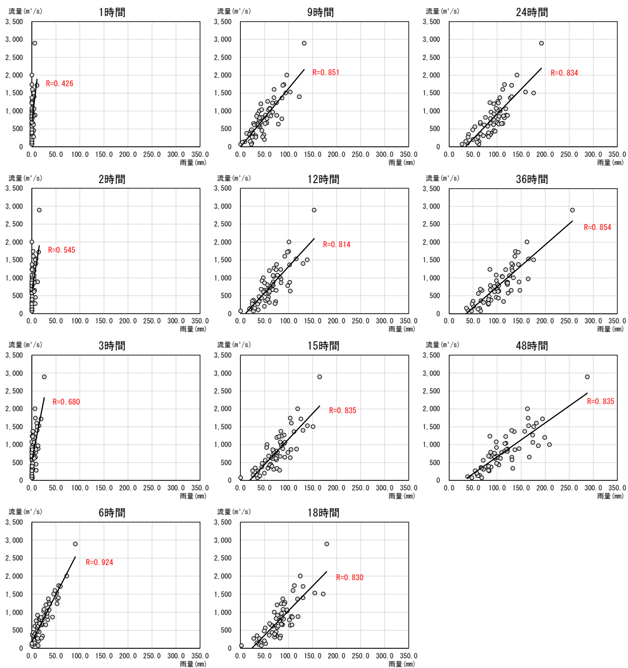
図 1-10 (2) ピーク流量と流域平均雨量の相関図 基準地点山手【定義②】
