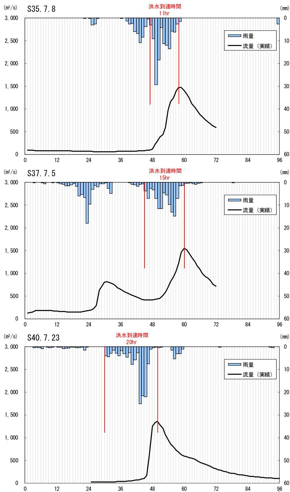
図 1-8(1) Kinematic Wave 法による洪水到達時間の検討
