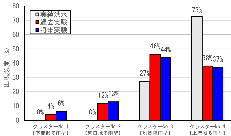
図 1-20 芦田川流域における実績洪水の降雨波形及びアンサンブル予測降雨波形の出現頻度 (クラスターごと)
