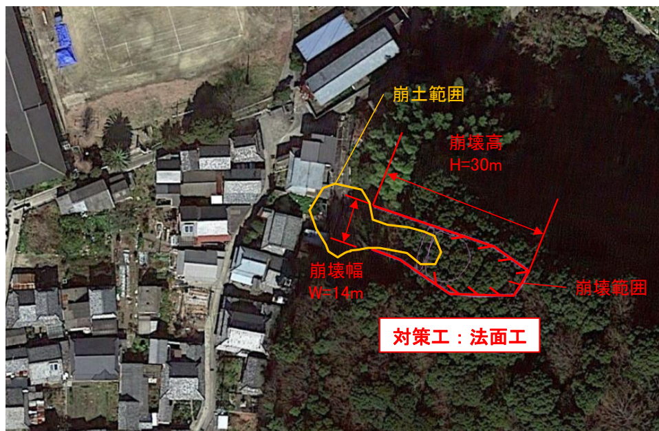
②斜面崩壊状況
