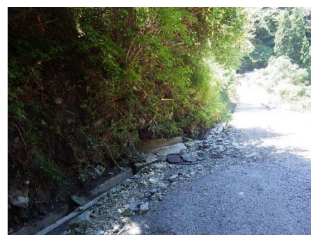
③押し出しによる側溝の変形
