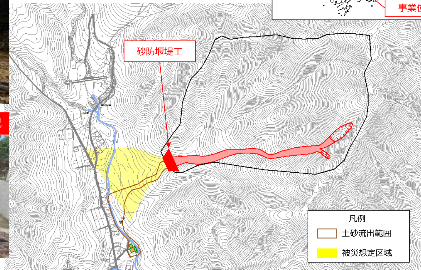
土砂流出状況
