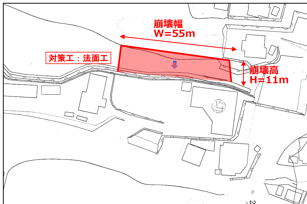
斜面崩壊状況
