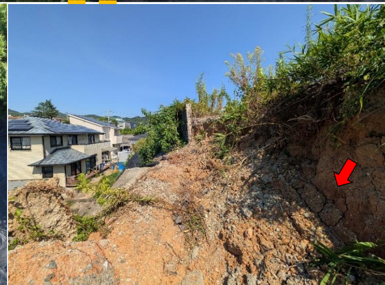
斜面の崩壊状況(滑落崖)
