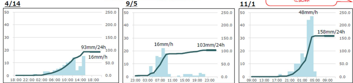
降雨状況 綾里川ダム雨量観測所 (県)
