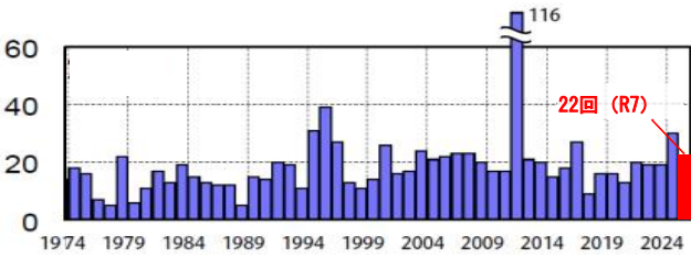
マグニチュード6.0以上の地震観測回数の推移
