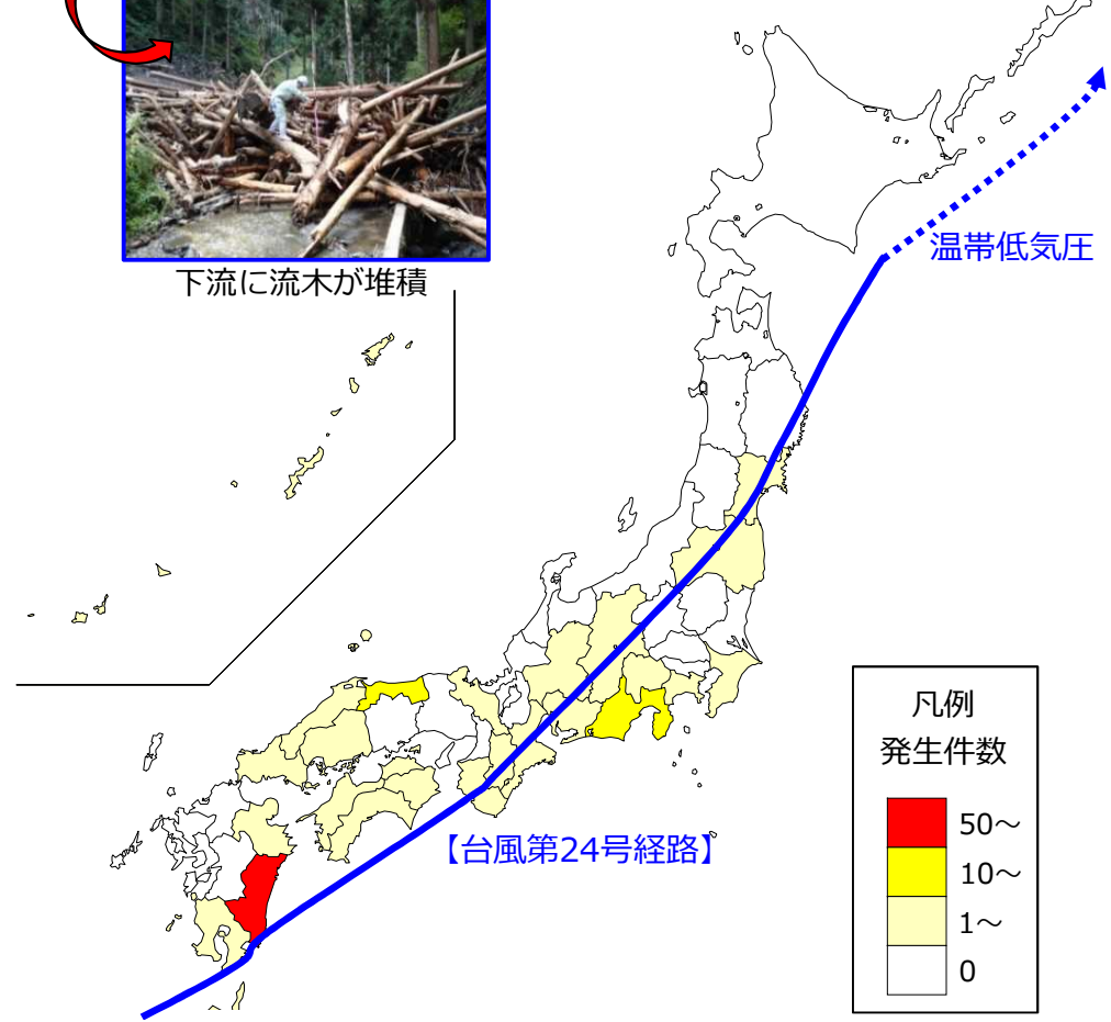
10/1 がけ崩れ
