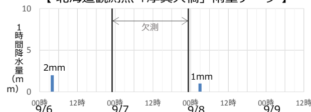
【北海道観測点「厚真大橋」雨量データ】
