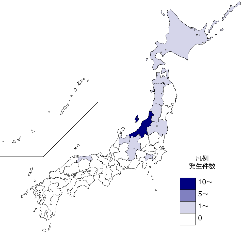
3/9 がけ崩れ
