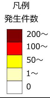
3/10 地すべり
