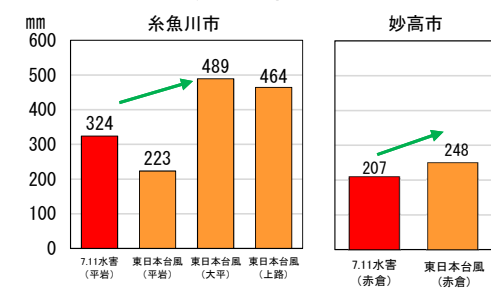
(1) 降水量の比較(24時間雨量)
