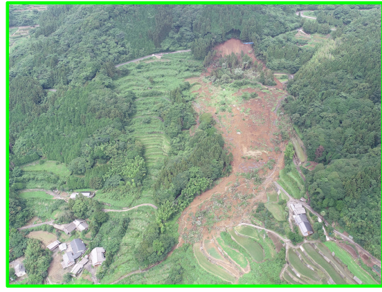
7/8 地すべり
