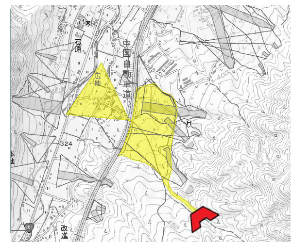
土砂を捕捉した砂防堰堤 警戒区域内の保全家屋16戸
