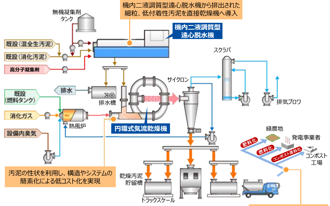
図 脱水乾燥システムのフロー
