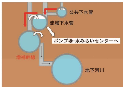
増補幹線と地下河川の関係図
