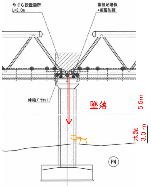
【正面図】
