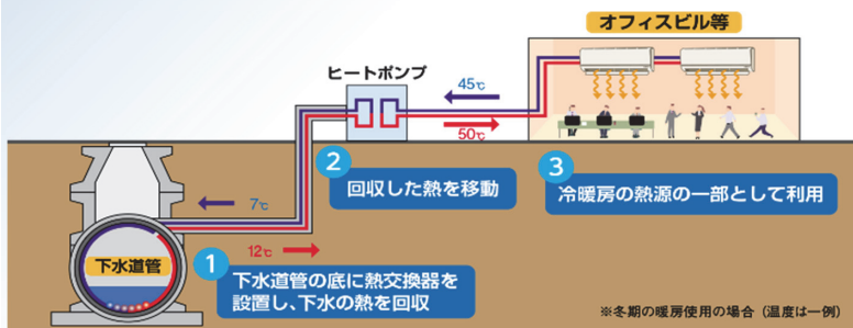
下水道管からの熱利用イメージ図
