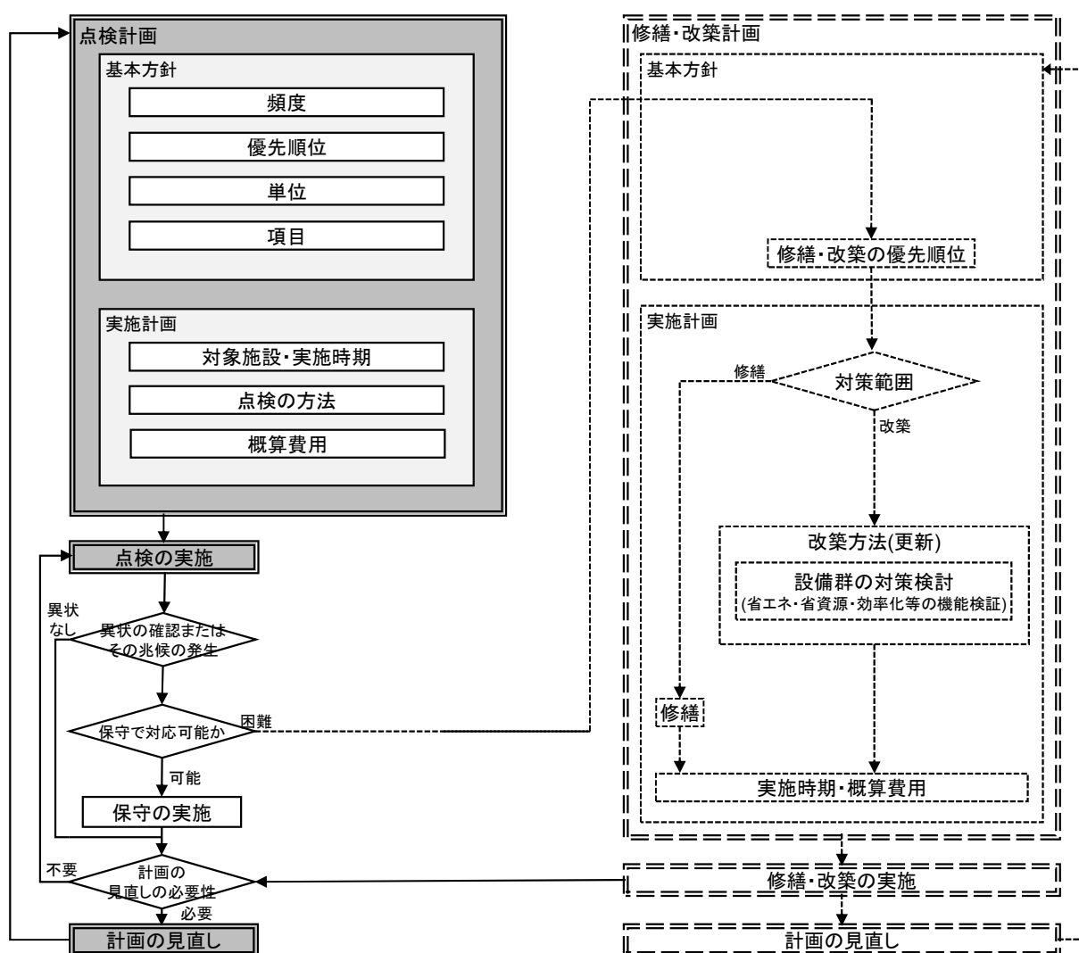
図 2-45 事後保全設備の点検の実施フローの例
