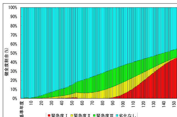
図 2-13 緊急度の推移（シナリオ4）
