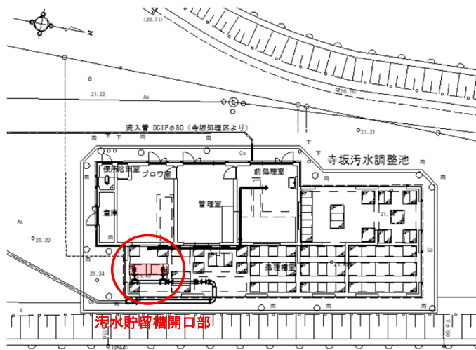
【状況平面図】
