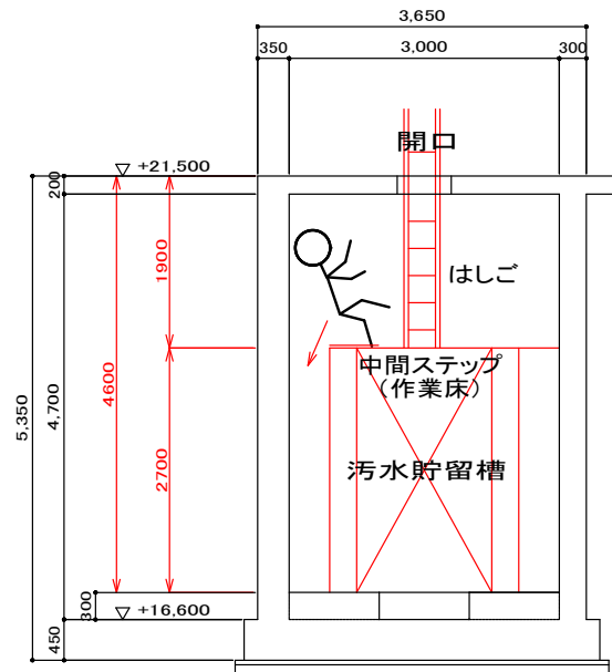
【状況断面図】
