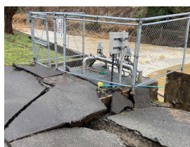
浄水場取水口の損傷
