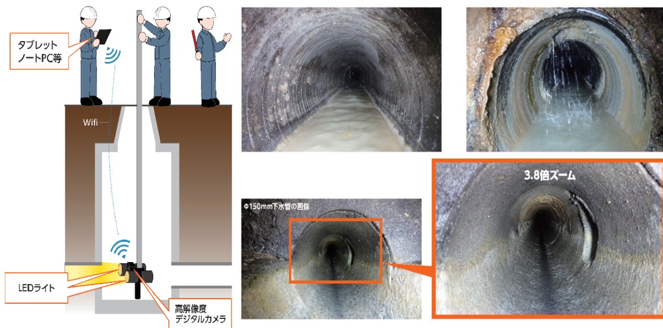
管口カメラの例
