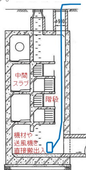
大口徑・大深度のマンホール例
