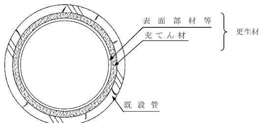
複合管の概念
