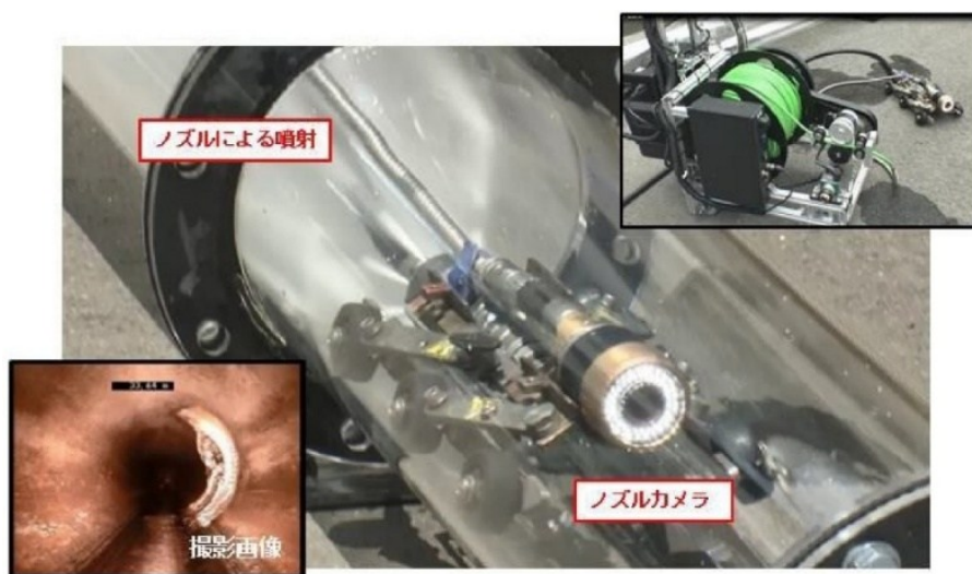
洗浄一体型カメラ（ノズルカメラ）の例
