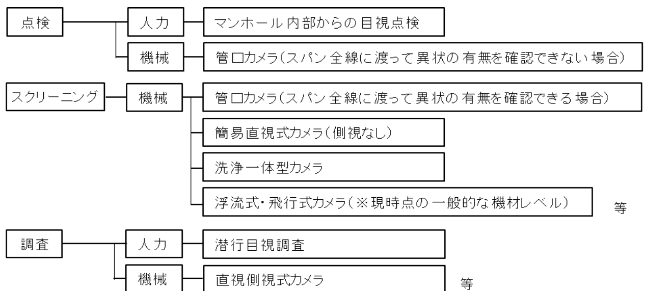
調査・スクリーニング・点検に関する手法・技術の分類（参考）（案）
