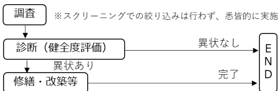
「重要管路」及び「枝線の要注意箇所」における手順
