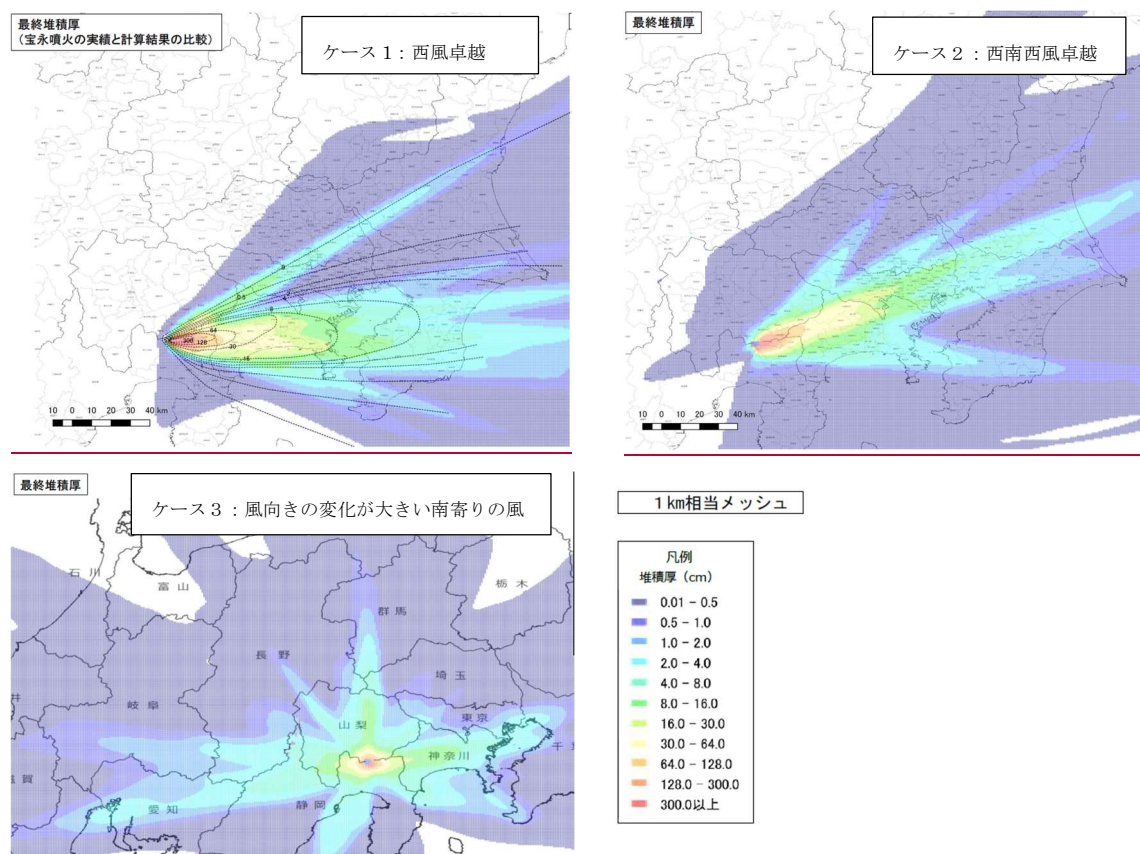
図 6-4-6-4 風向・風速の違いによる降灰分布図（富士山の例）
