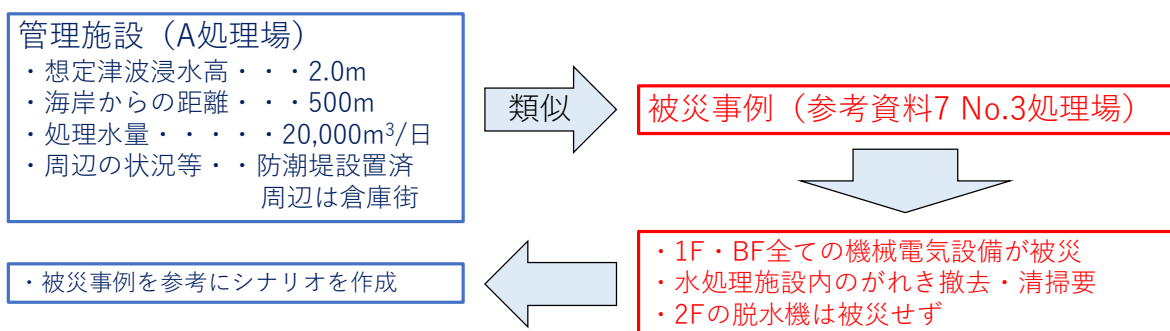
図 2-8-2-7 被害想定イメージ（津波）
