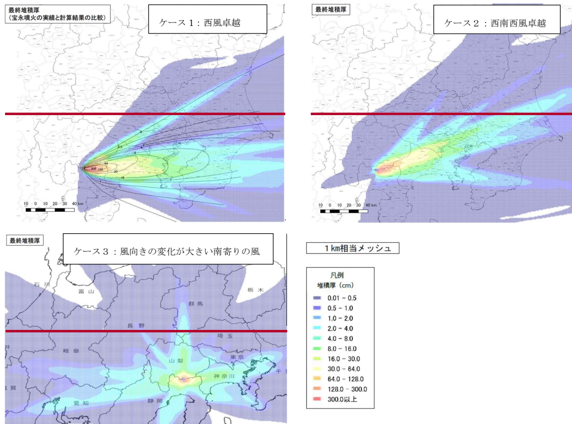
図 3-16 風向・風速の違いによる降灰分布図（富士山の例）
