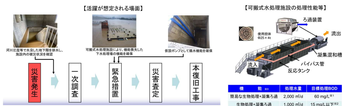
図 4-8 活用が想定される場面と可搬式水処理施設の概要
