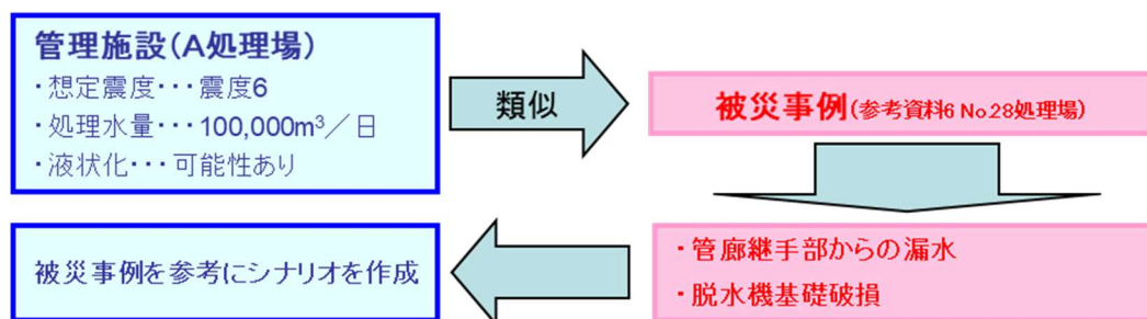
図 2-7 2-6 被害想定イメージ（地震）
