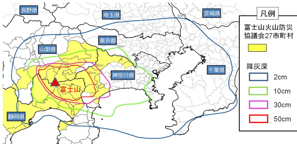
図 6-2 6-2 降灰範囲と火山防災協議会市町村の位置関係（富士山の例）
