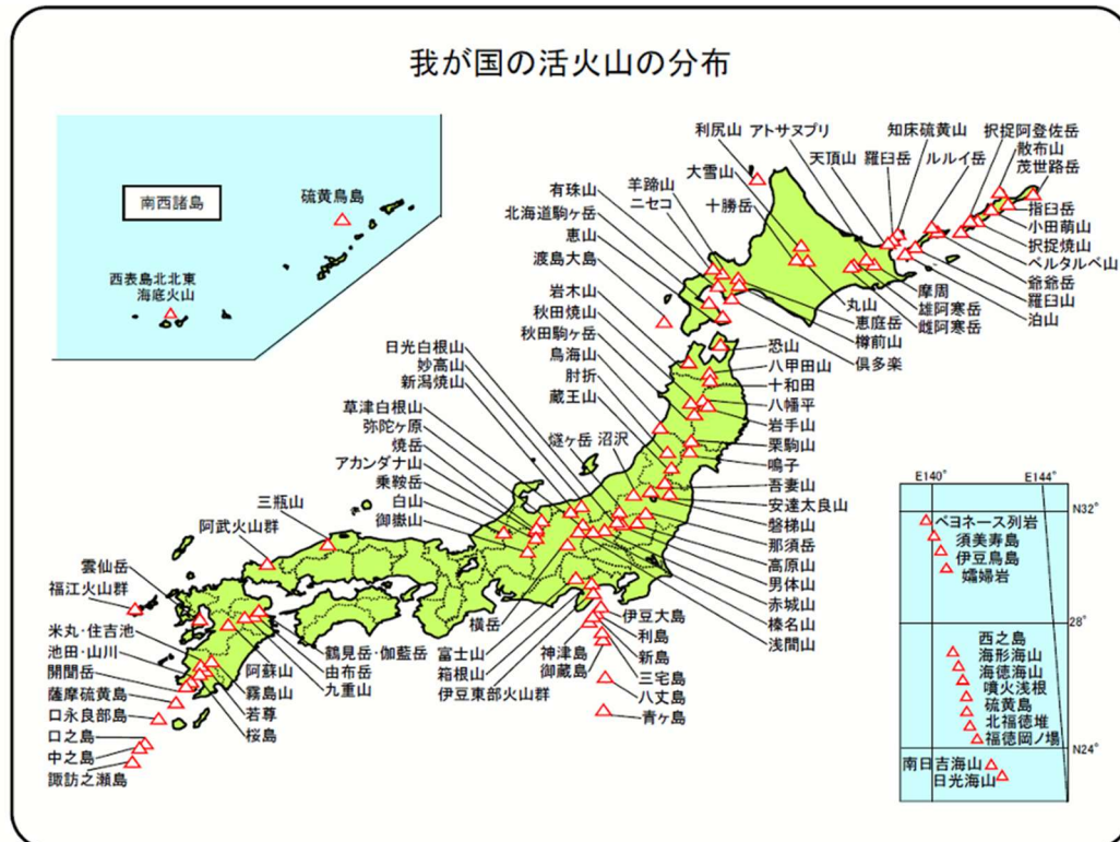
図 6-1 6-1 111 の活火山の分布
