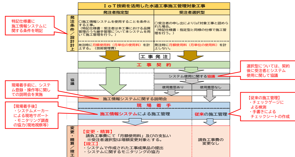
【施工情報システムを使用した水道工事のフロー図】
