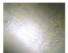
【異常なし】 モルタルライニング健全
