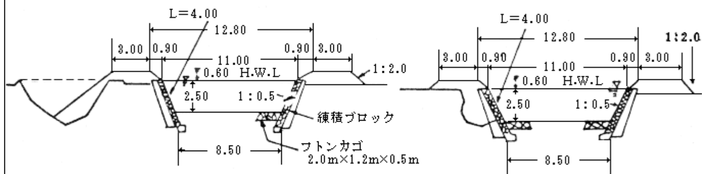
A-A'断面
