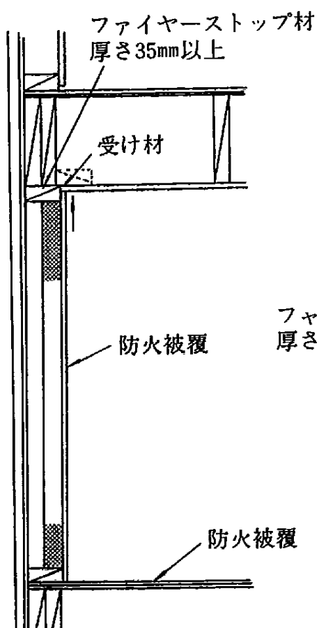
壁と床の接合部
