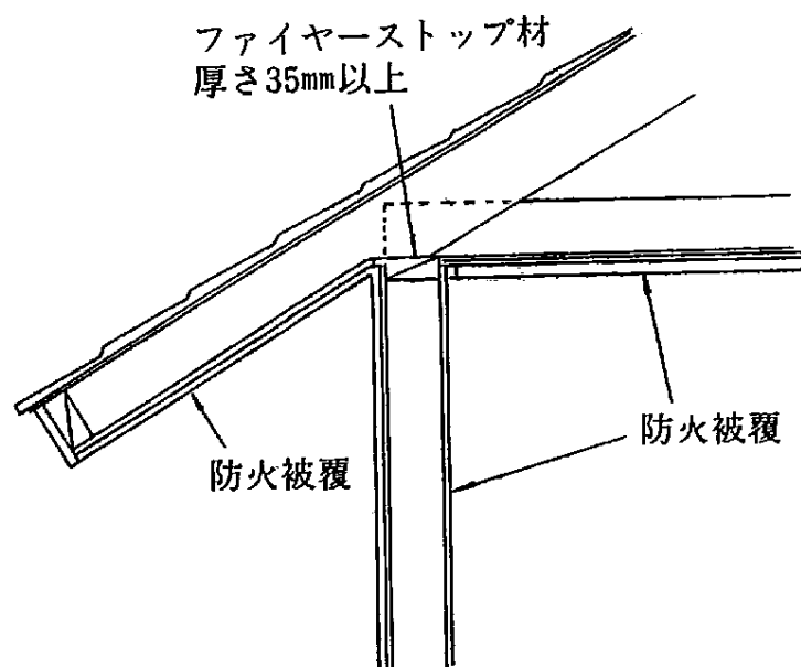
壁と屋根の接合部
