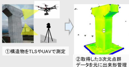
3次元測量等を活用した出来形管理の効率化
