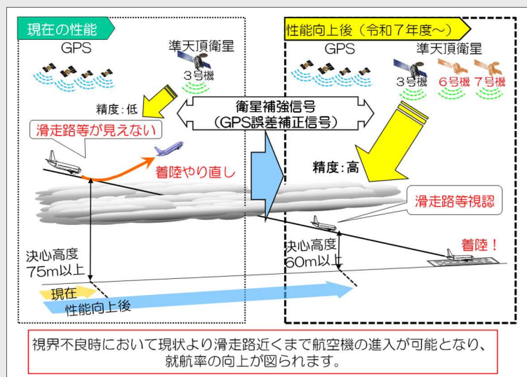
準天頂衛星システムを利用した衛星航法システム(SBAS)
