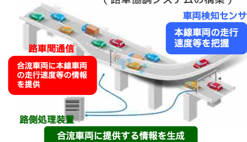
▲インフラ側からの情報提供事例 (高速道路の合流部において、本線の交通状況をセンサで検知し、自動運転車に情報提供)
