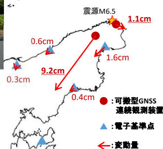
可搬型GNSS連続観測装置が捉えた地殻変動 (令和5年5月石川県能登地方の地震)
