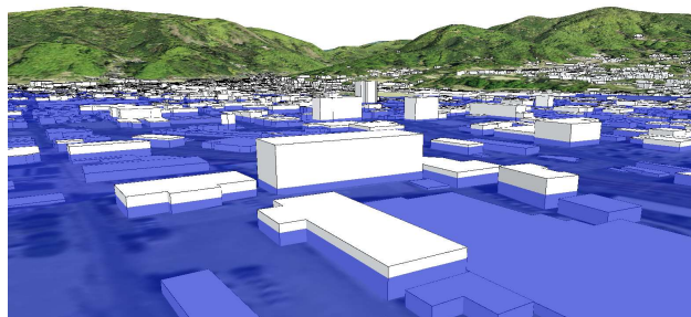
3次元地図による地形や建物を考慮した 詳細な浸水シミュレーションへの活用
