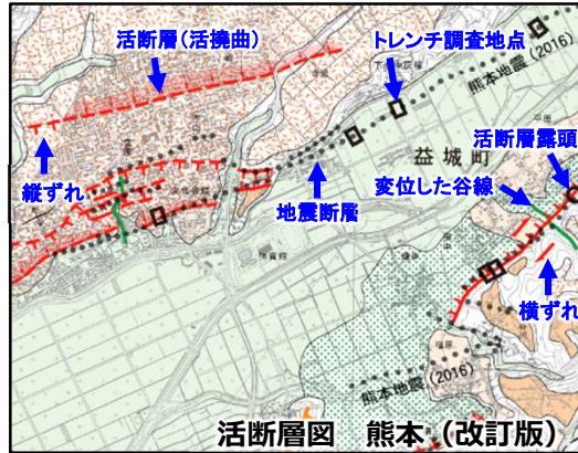
右横ずれした地震断層 (平成28年(2016年)熊本地震)
