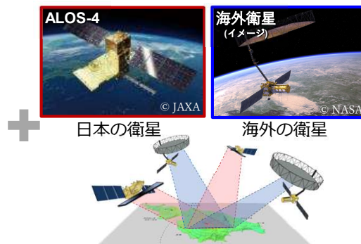
地表面の動きを面的に把握できる衛星SARで、複数の衛星データを用いて3次元解析
