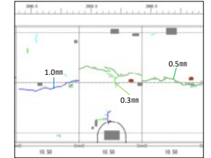
変状展開図
