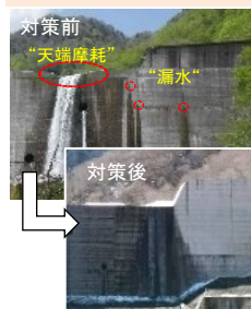
砂防堰堤の改築
