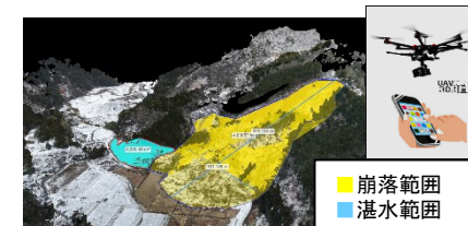
▲①UAV空撮画像から作成した3次元モデル
