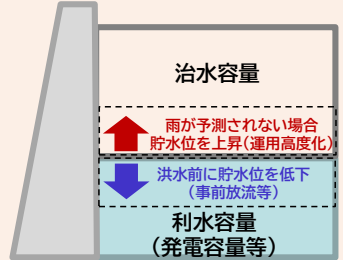
ハイブリッドダムのイメージ
