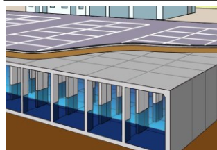
雨水貯留施設
