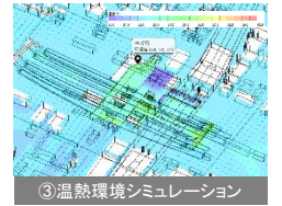
③温熱環境シミュレーション
