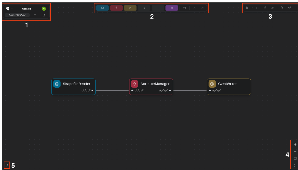
図 エディタの画面構成
