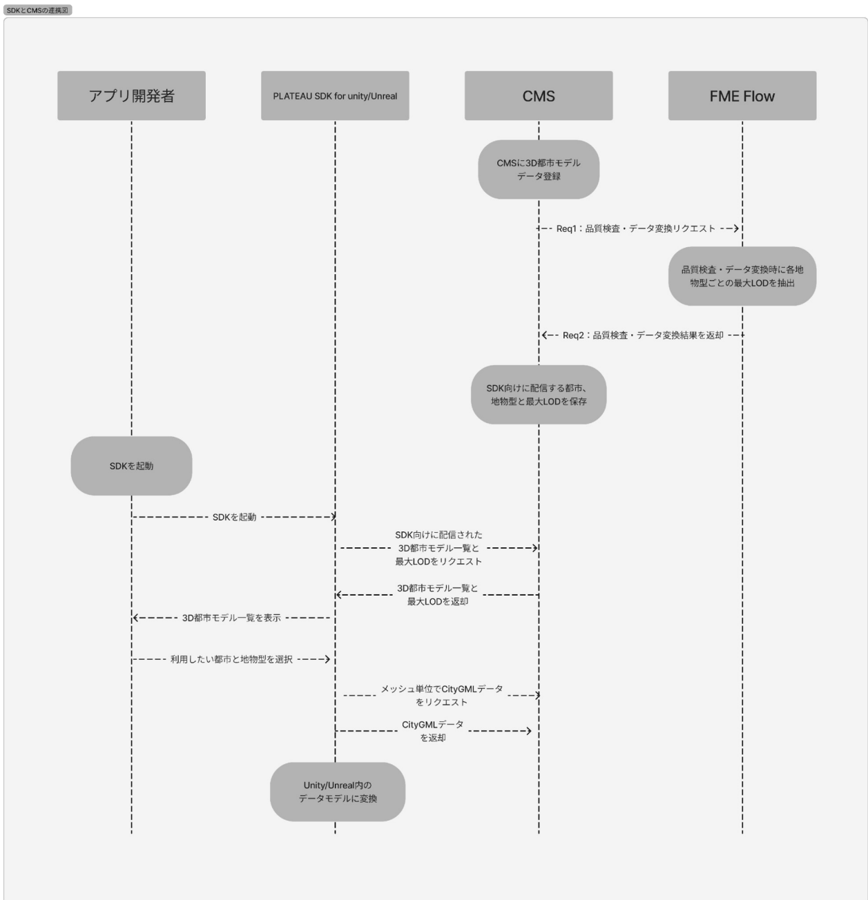
図 複数システム連携図
