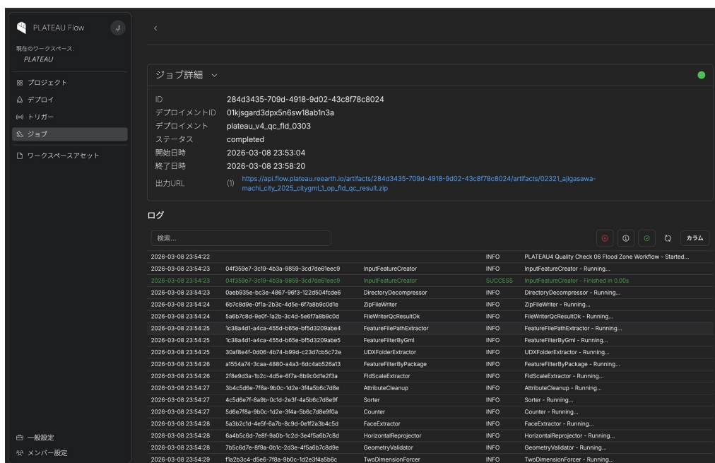
図 ジョブ詳細ページ
