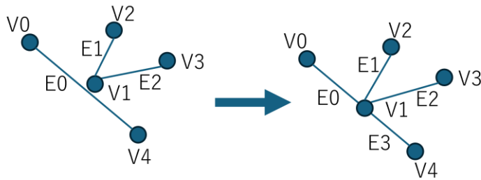
図3-1-51 辺と頂点の距離による分割
