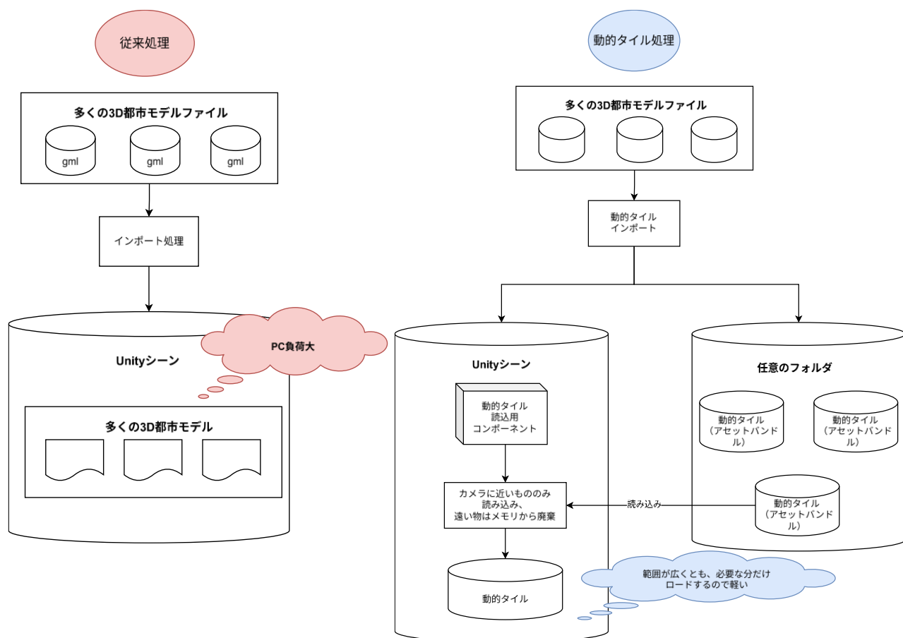
図3-1-21 ゲームシーンに直接配置する処理と動的タイル処理の違い
