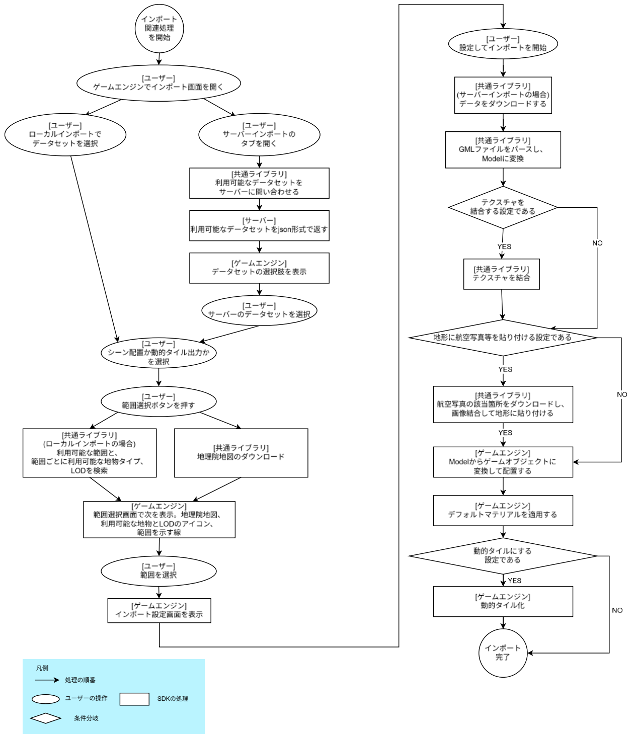
図3-1-3 インポート処理の概要
