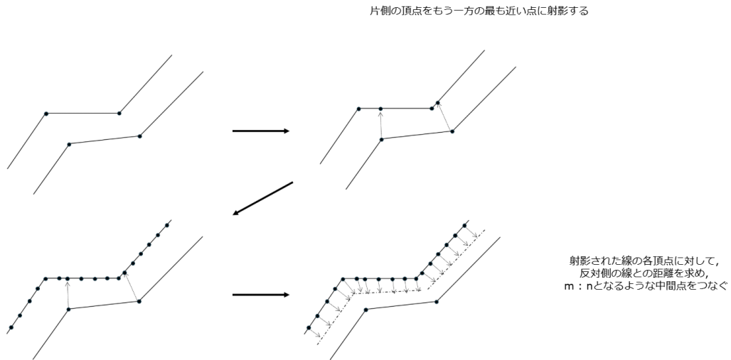
図3-1-59 車道分割の概略
