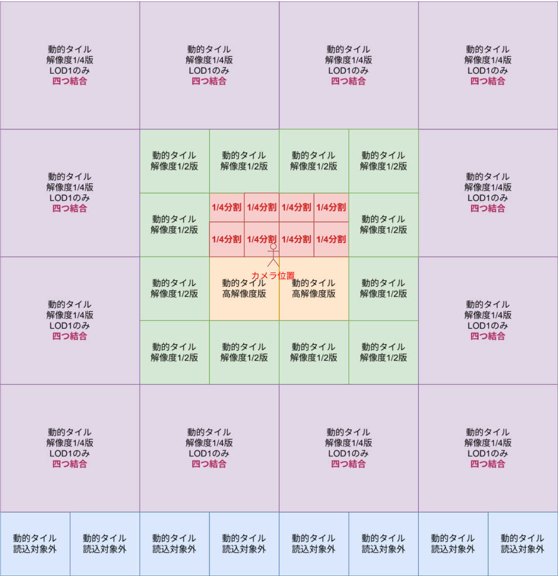
図3-1-22 タイル処理の図
