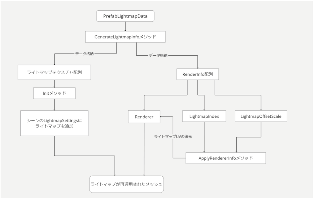
図3-2-57 ライトマップの適用イメージ
