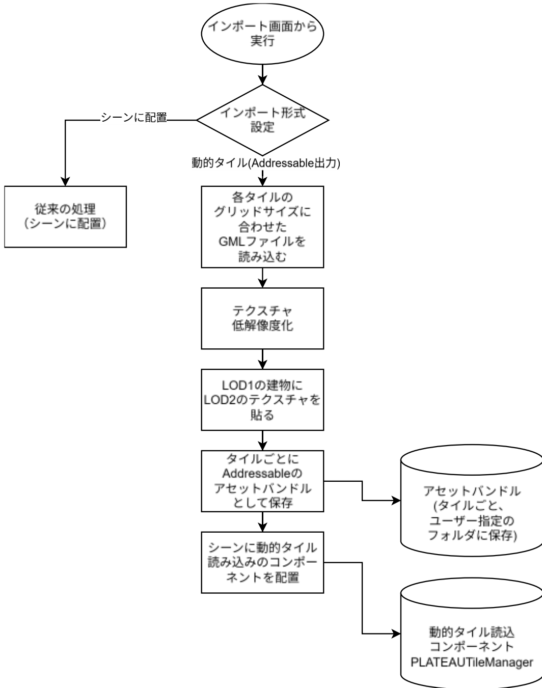
図3-1-23 動的タイルの処理の流れ
