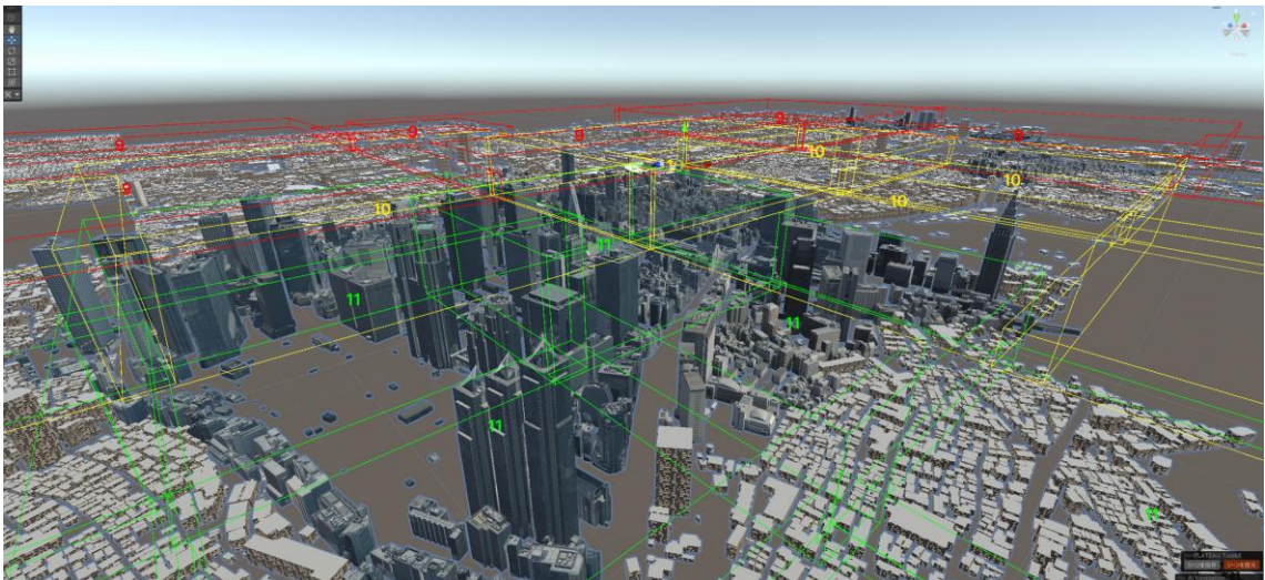
図3-1-20 動的タイルを適用した新宿区の3D都市モデルに 詳細度を重ねて表示した例
