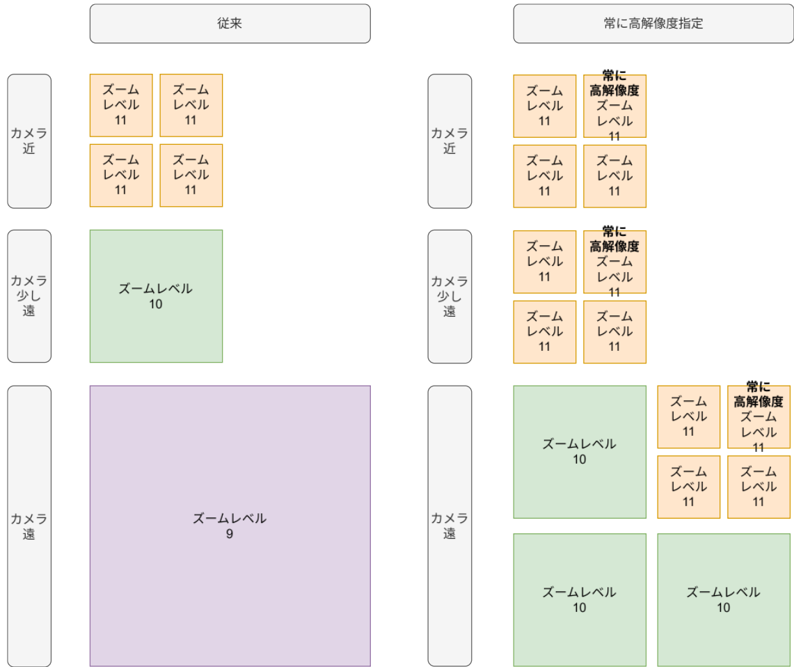
図3-1-26 「常に高解像度で表示するタイル」によるタイルの敷き詰め方の変化
