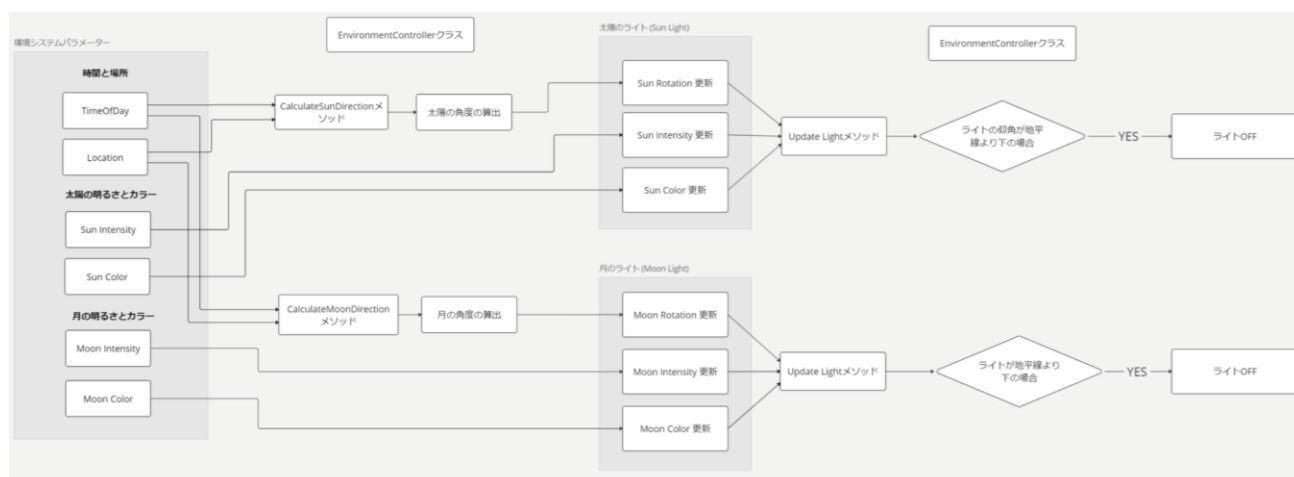
図3-2-33 時間の変更アルゴリズム
