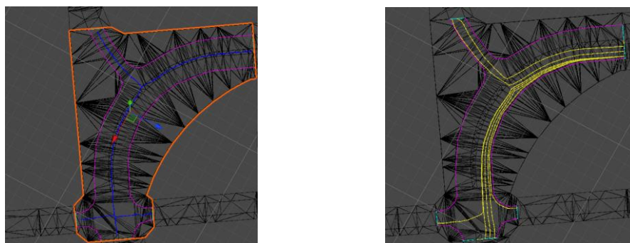
図3-1-62 ボロノイ図による中央を通るパス（左図） スプライン計算の結果（右図）
