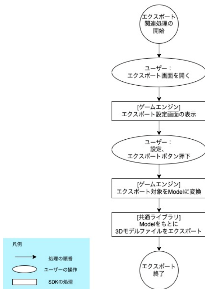
図3-1-27 エクスポート処理の流れ
