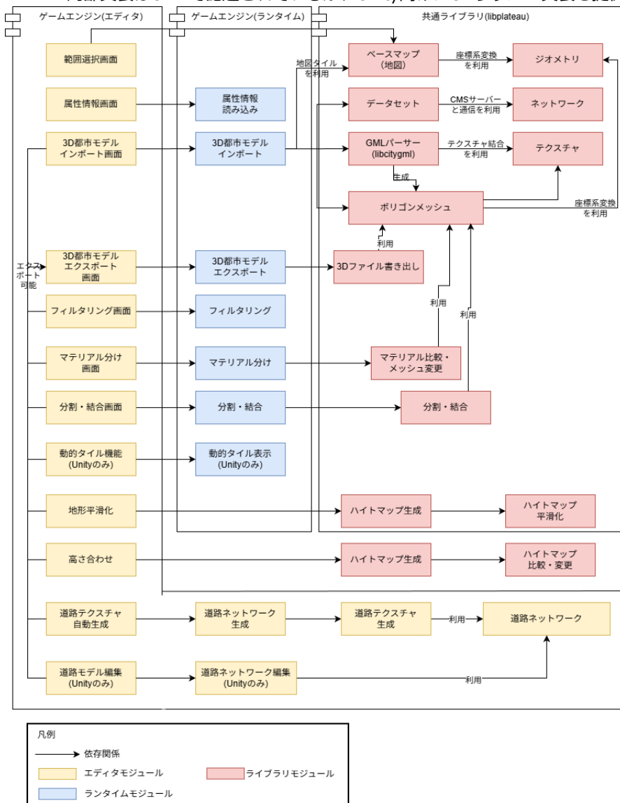
図1-1-3 PLATEAU SDK for Unity/Unrealのアーキテクチャ
