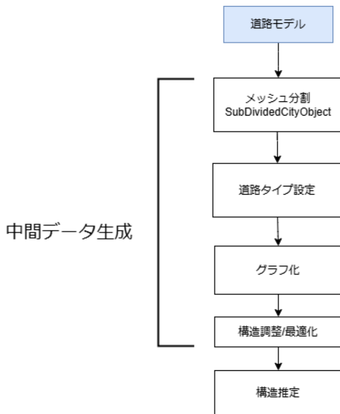
図3-1-45 道路ネットワーク推定フロー
