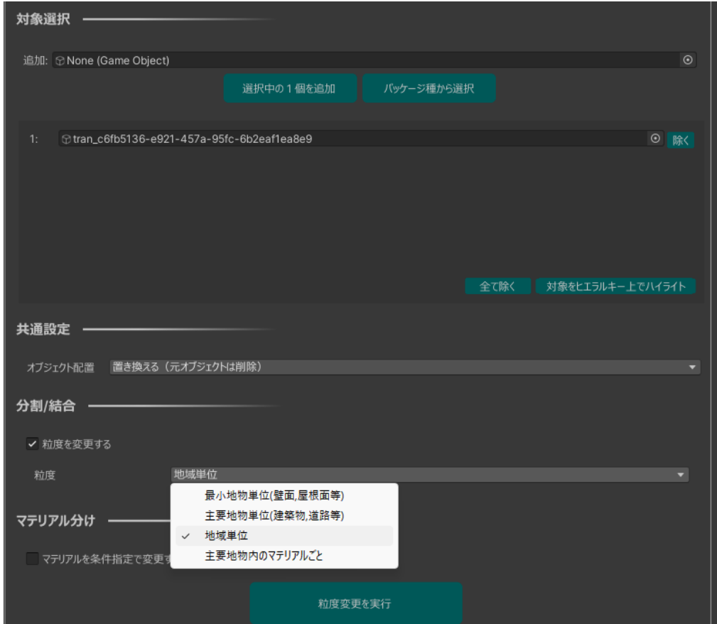
図3-1-34 分割結合画面
