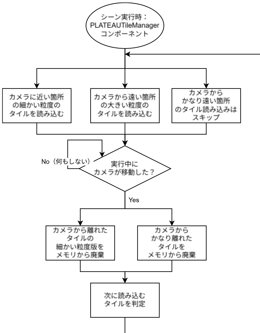
図3-1-24 動的タイルをゲーム中に読み込む処理の流れ
