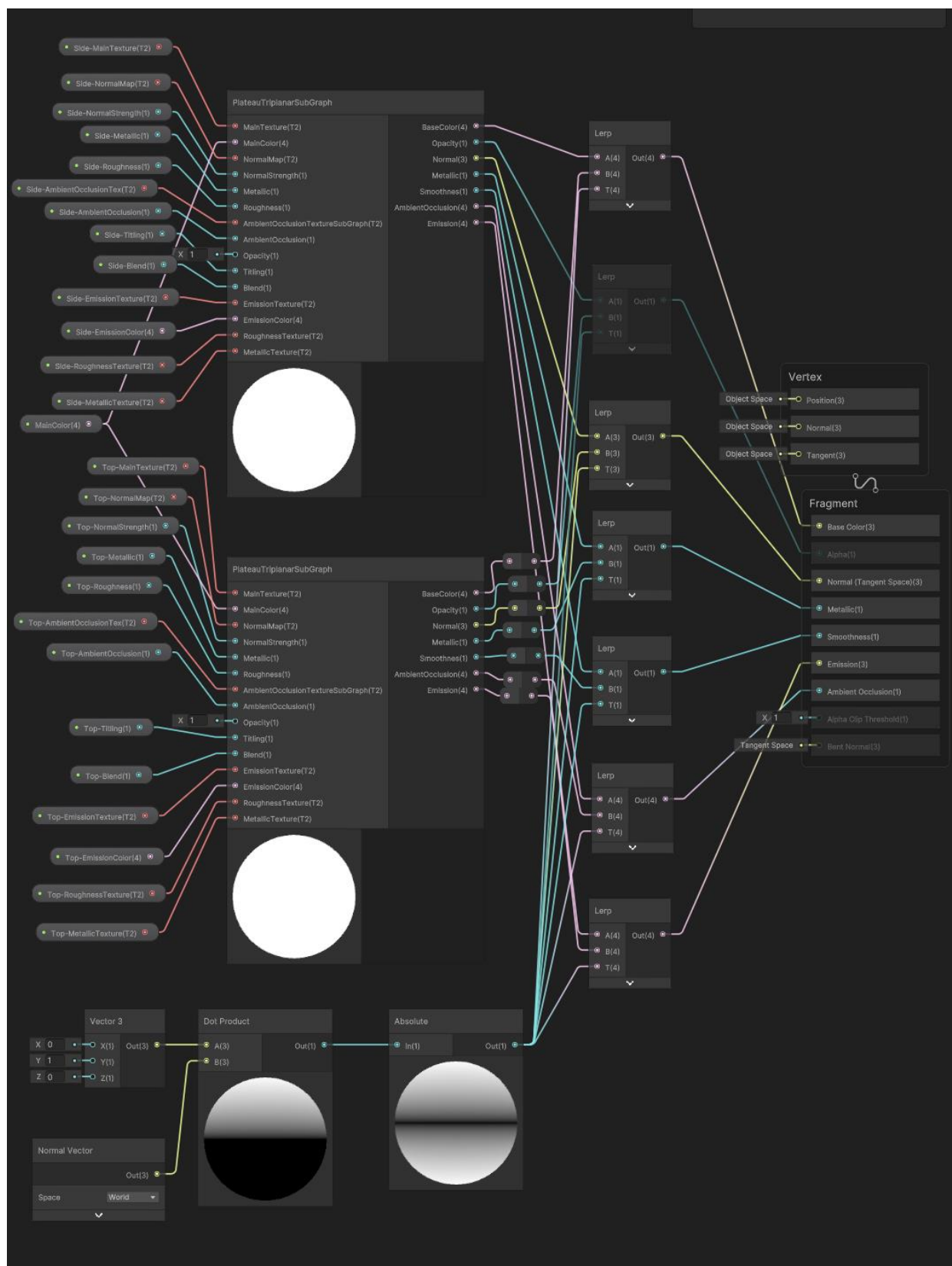
図3-1-16 PlateauTriplanarShader(DualTextures)の実装
