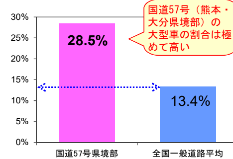
図2 国道57号の大型車混入率
