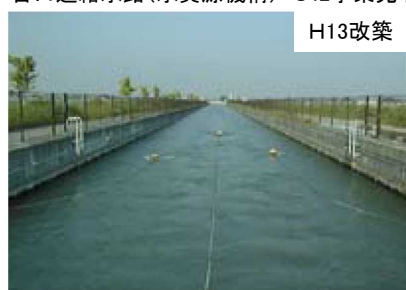
合口連絡水路(水資源機構) S42事業完了
