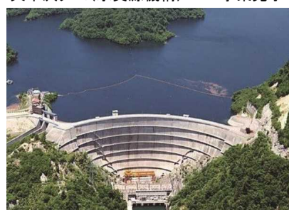
利根大堰(水資源機構) S42事業完了 H9改築
