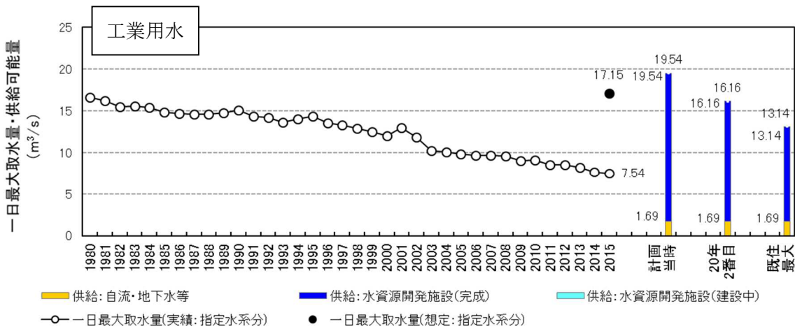
図 28 指定水系に依存する水道用水の需要実績・想定と供給可能量の比較
