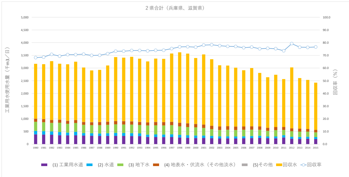
図 20 工業用水使用水量、回収率の推移 (フルプランエリアのうち、滋賀県、兵庫県 の 2 県の合計 (大阪府を除く))
