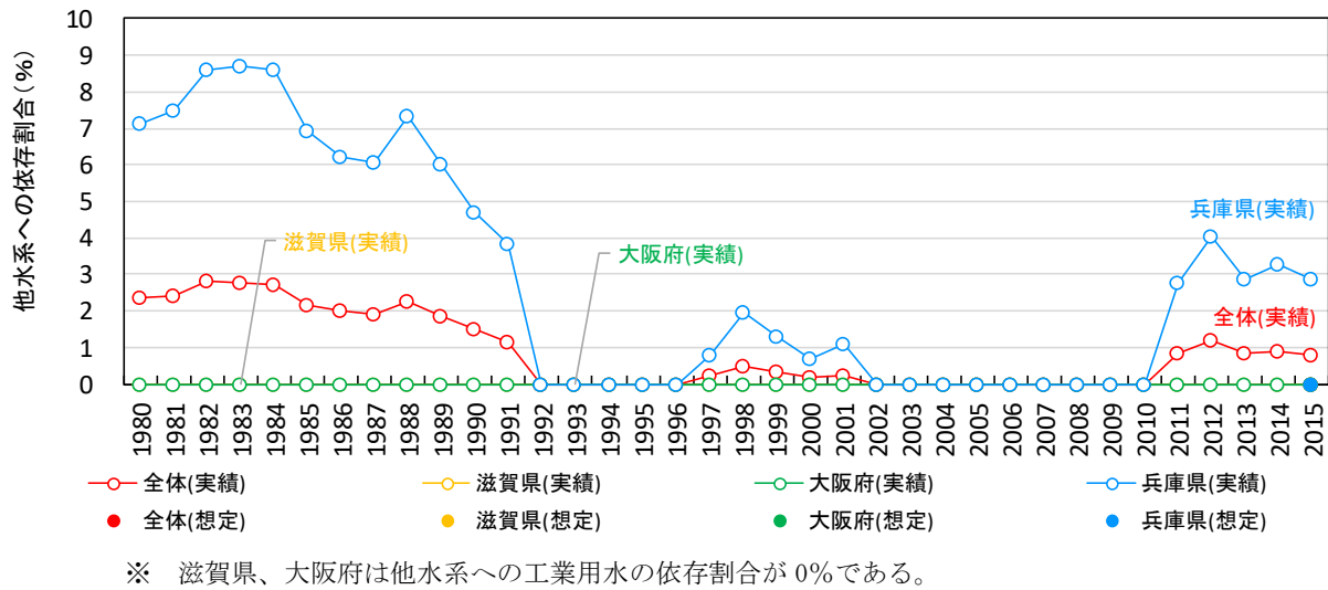
図 23 工業用水 各府県における一日最大取水量の他水系への依存割合の推移
