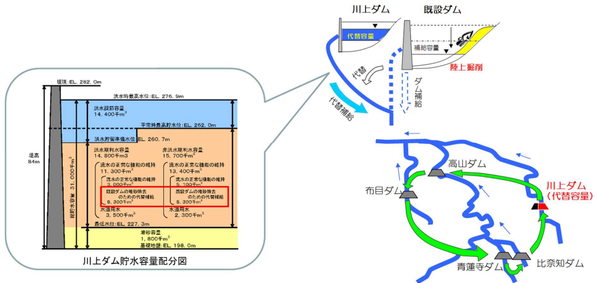
図 62 木津川上流ダム群の堆砂対策（川上ダムによる代替補給イメージ図）
