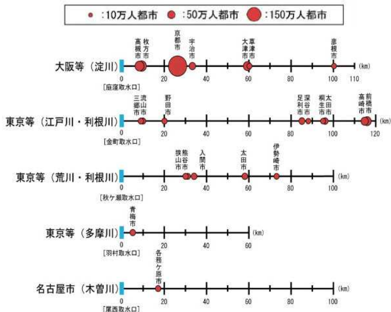
図 56 大都市の主要取水地点と上流都市の関係
