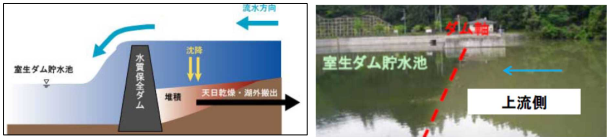
図 72 室生ダムにおける水質保全設備 副ダム
