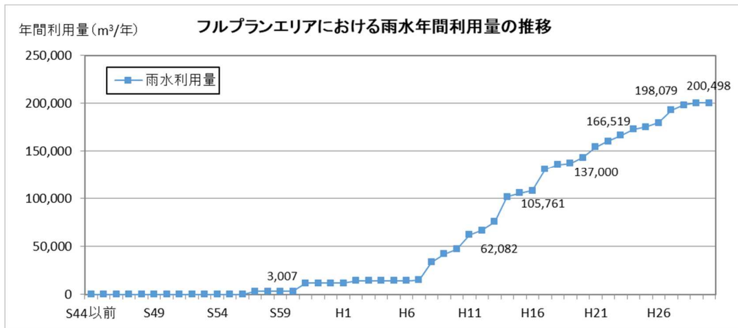
図 54 フルプランエリアにおける雨水年間利用量の推移
