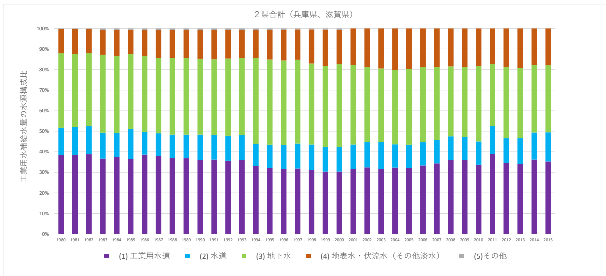
図 21 工業用水補給水量の水源構成比の推移 (フルプランエリアのうち、滋賀県、兵庫県 の 2 県の合計 (大阪府を除く))
