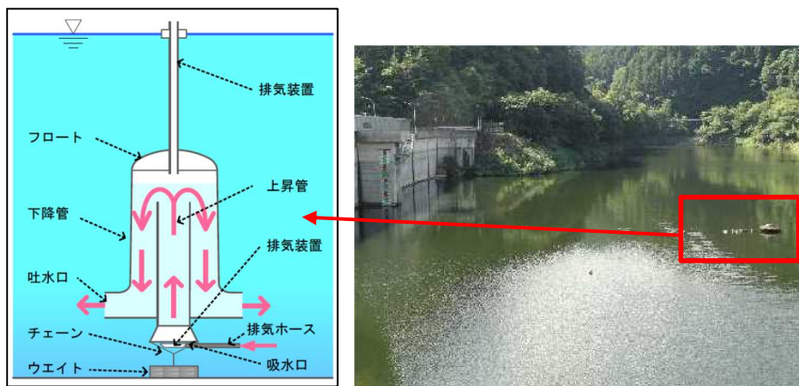
図 69 高山ダムにおける水質保全設備 曝気循環装置
