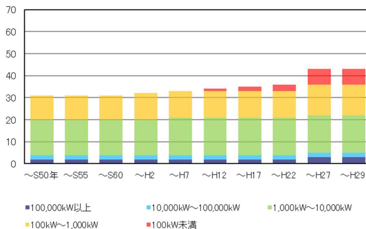
図 41 指定水系（一級河川）における水力発電所設置箇所数の推移
