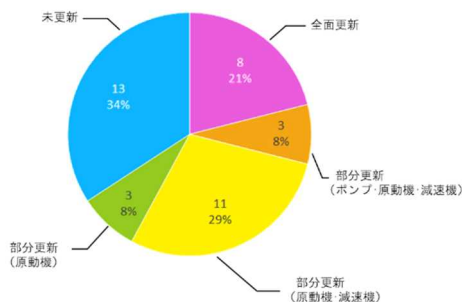
排水機場の更新実態 (設置後50年以上経過 N=38)
