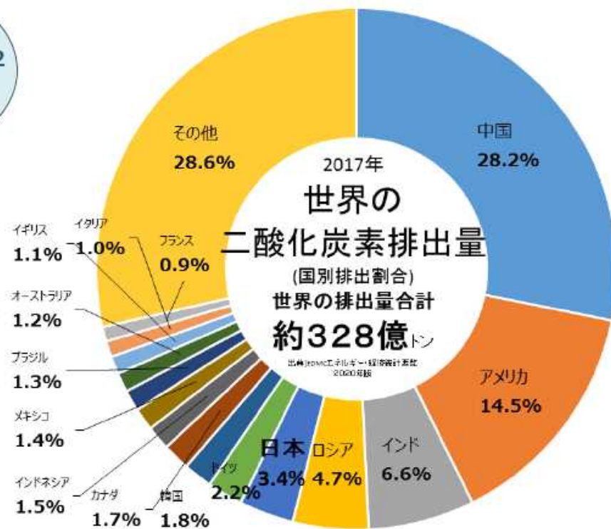
世界のエネルギー起源CO2排出量 (2017)
