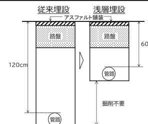
美深町の凍結深さを 考慮した浅層埋設のイメージ
