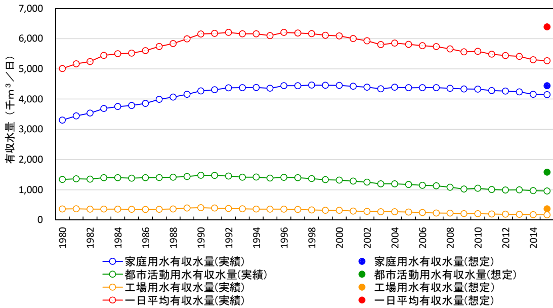
参考図表 3 下水道における有収水量の推移
