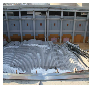
体育館の屋根崩落被害(埼玉県)
