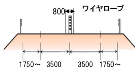
（土工部の横断面図）
