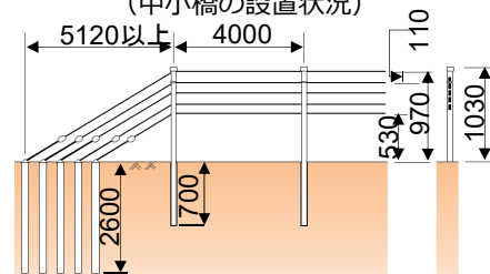
（土工部の縦断面図）
