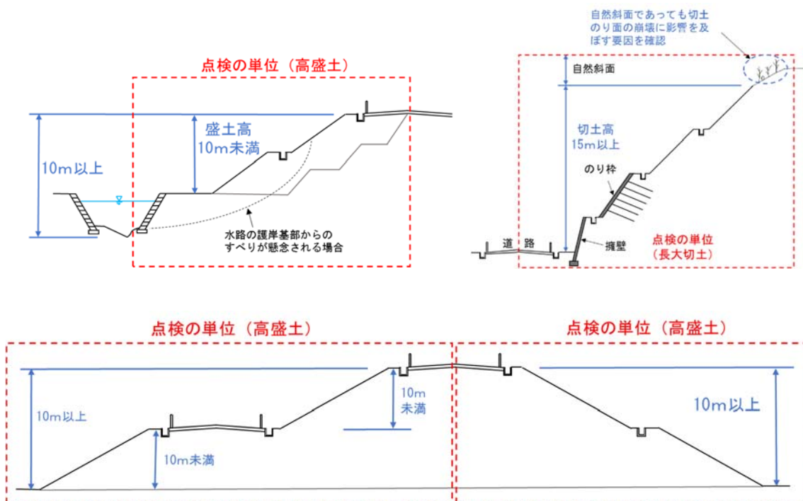
図－３ 特殊な長大切土、高盛土の例
