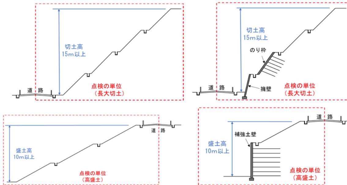
図－２ 長大切土、高盛土の例
