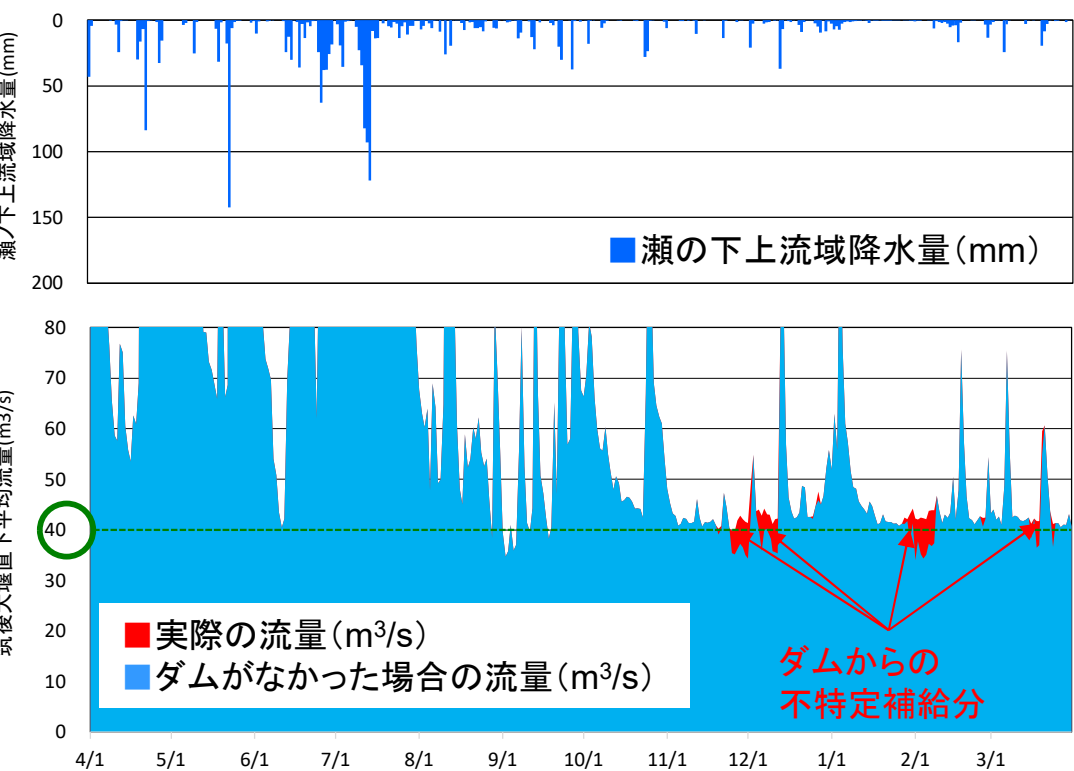
松原・下釜ダムによるノリ期の河川流量改善例 (H22)
