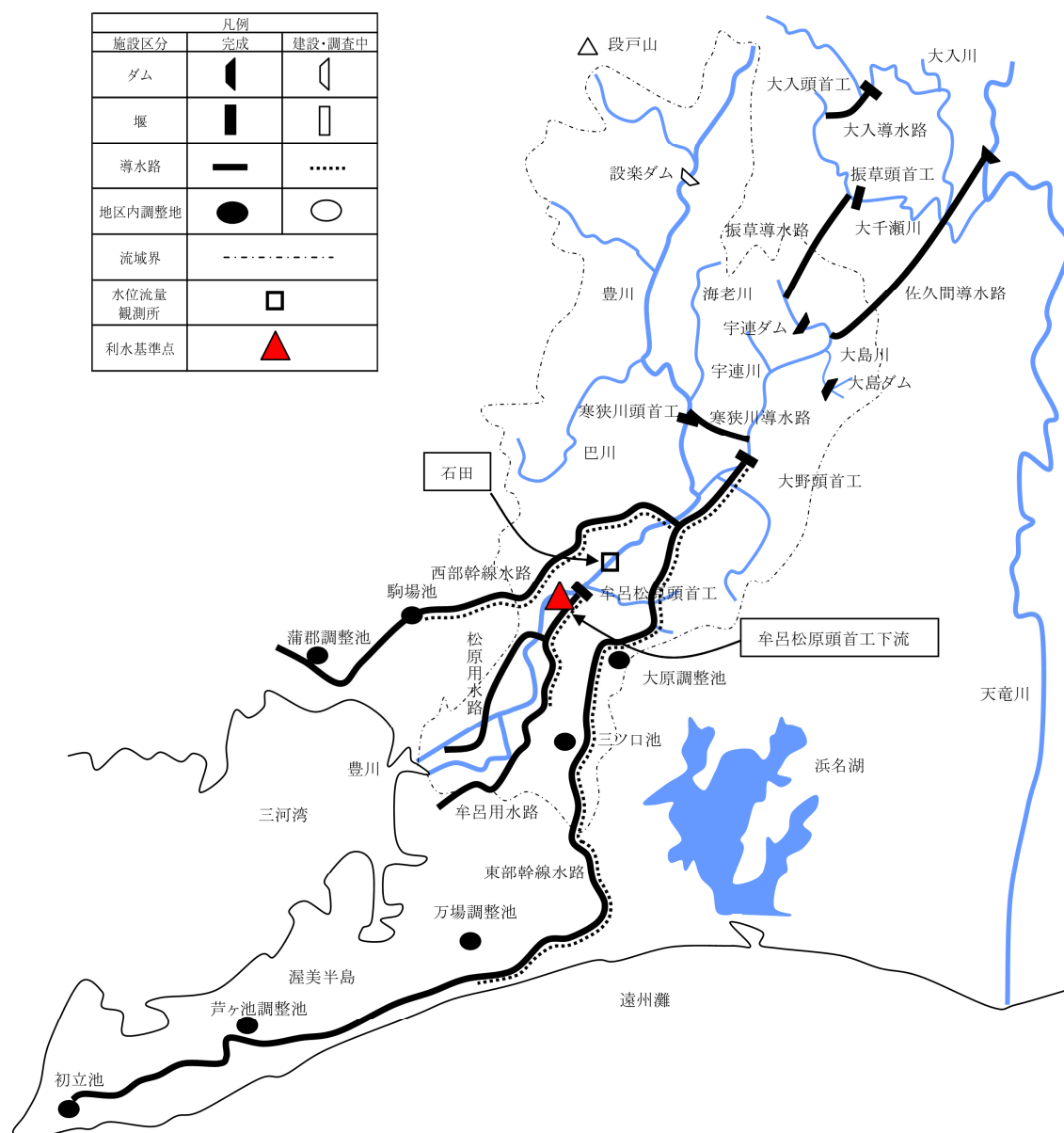
図 48 豊川水系利水計画位置図
