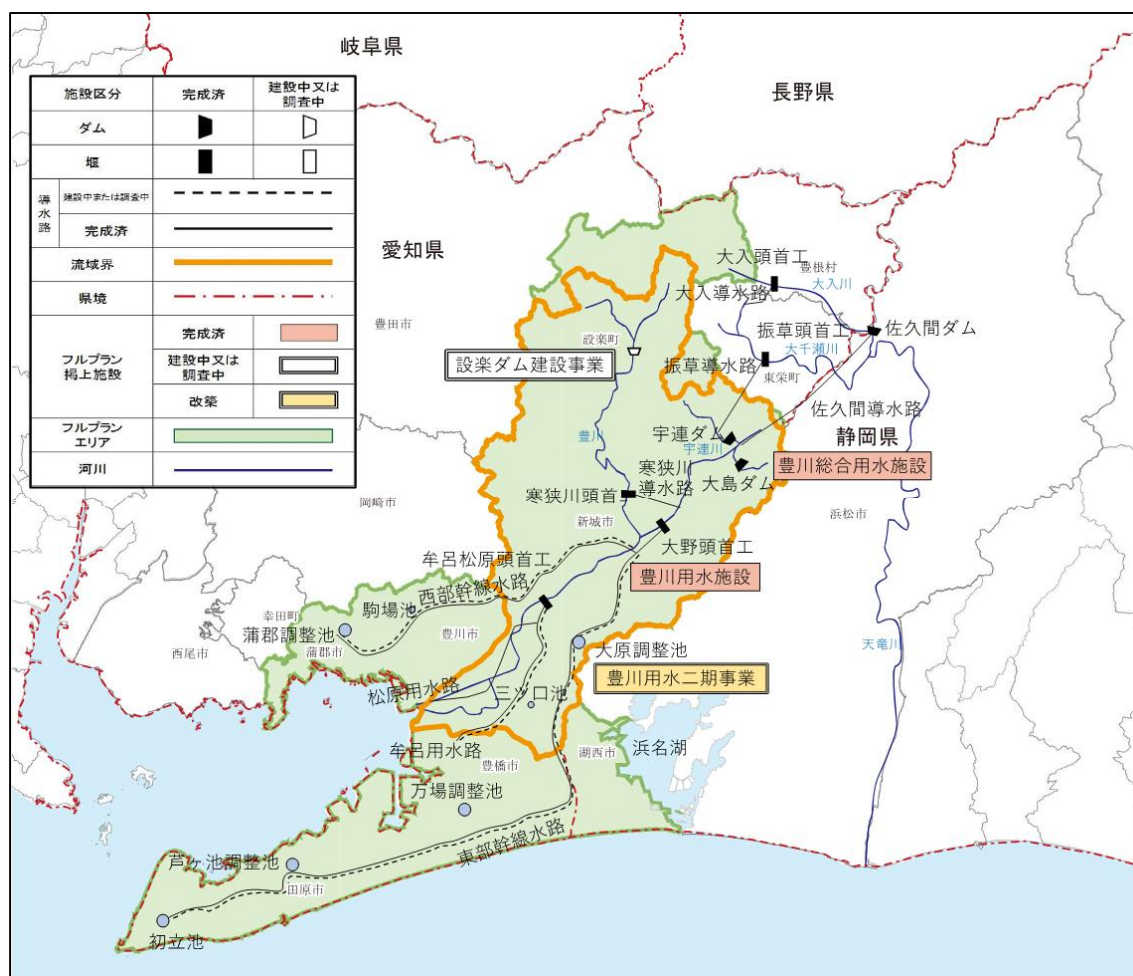
図 1 次期「豊川水系における水資源開発基本計画」のフルプランエリア
