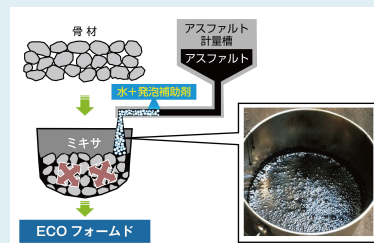
アスファルトの中温化技術
