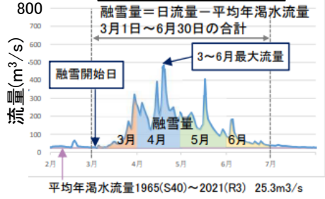
融雪量設定の考え方
