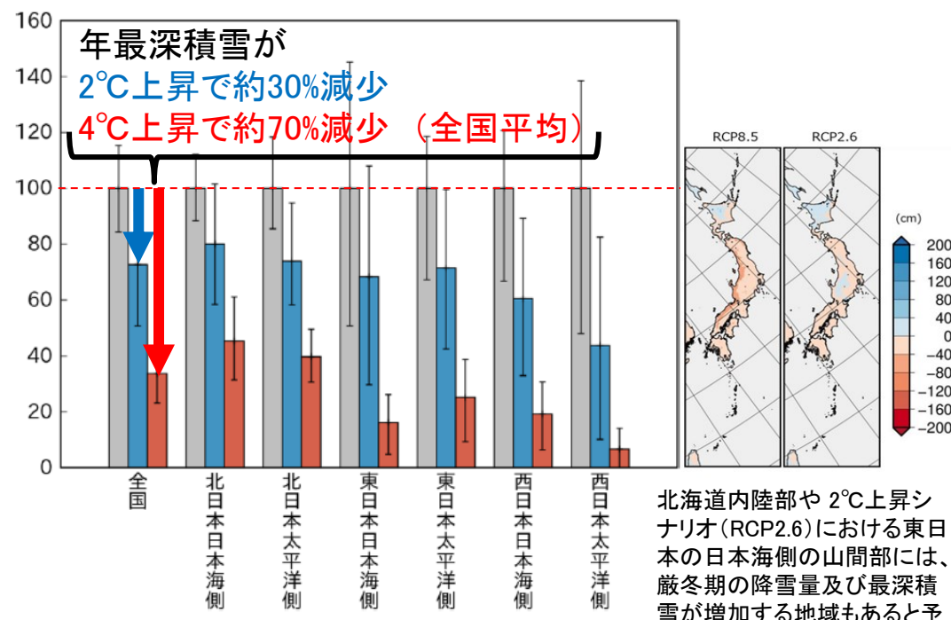
気候変動の影響による年最深積雪(%)
