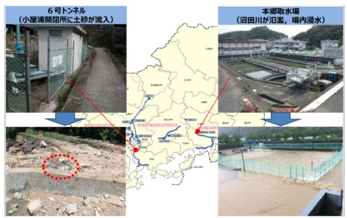
広島県工業用水の被災状況 1)
