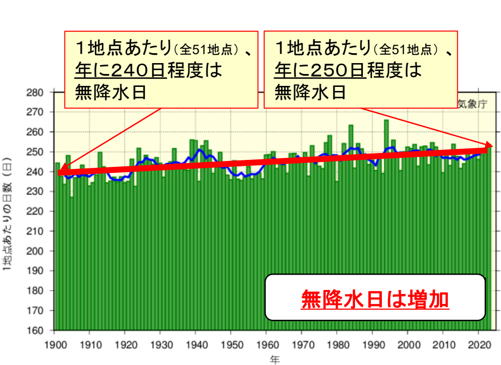
日降水量1.0mm未満の年間日数の経年変化(1901～2023年)
