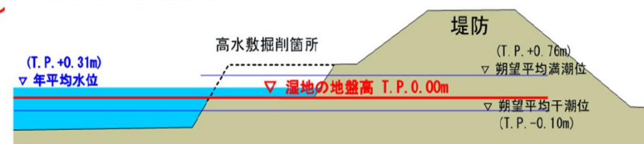
高水敷掘削箇所の状況(2006年12月)
