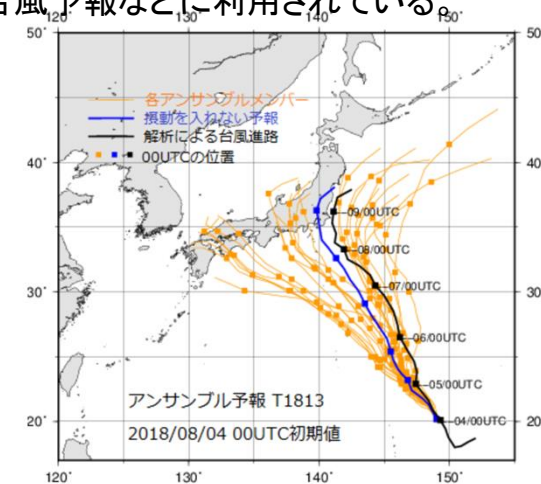
台風進路のアンサンブル予報の例 ※気象庁HPをもとに作成
