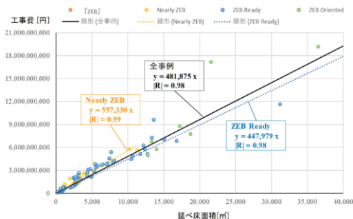
図-10: 延べ床面積 - 工事費
