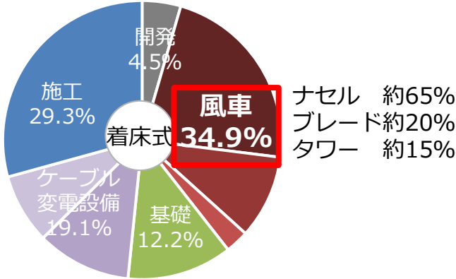
＜洋上風力のCAPEX構造＞
