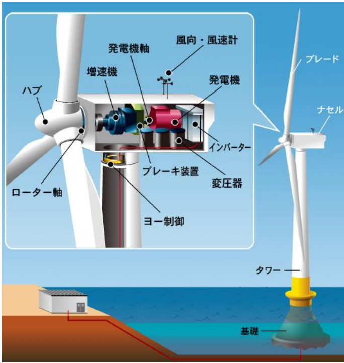
＜風車の構造＞
