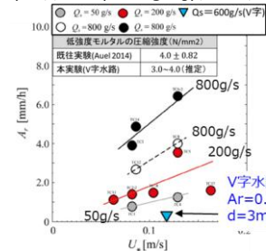
図-7 長方形断面との損傷速度の比較
