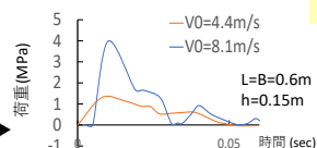
海氷の衝突力波形
