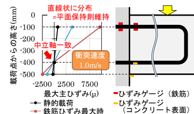
図-1 実大サイズのRC 載荷梁の衝撃载荷実験結果
