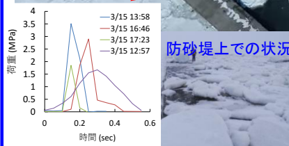
海氷の衝突力波形
