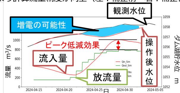
予測雨量に基づき事前放流することによる効果
