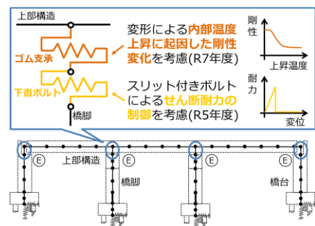
図-2 スリット付きボルト、ゴム支承の剛性変化を考慮した解析モデル
