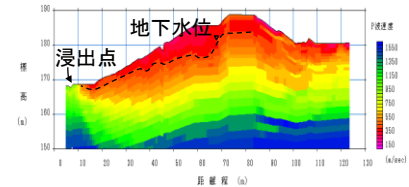
図-4 P波屈折法探査により把握した被災盛土内部の地下水位分布
