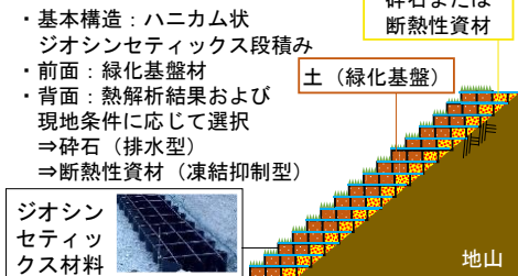
図-4 新たな複合型法面保護工の概要
