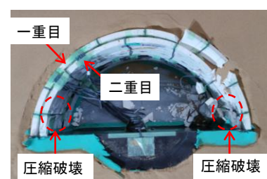
二重支保工の载荷実験
