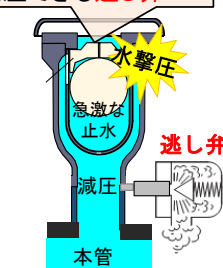
図3 空気弁における逃し弁の設置と作動時の模式
