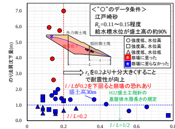
図-5 既設盛土への耐震対策の規模と盛土の沈下量の関係
