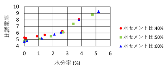
コンクリートの比誘電率（1GHz 帯域）
