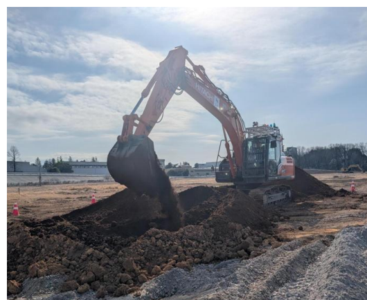
写真-1 掘削時データ取得実験状況
