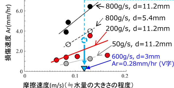
損傷速度Arの既往研究（長方形断面）との比較 Auel (2014)に加筆
