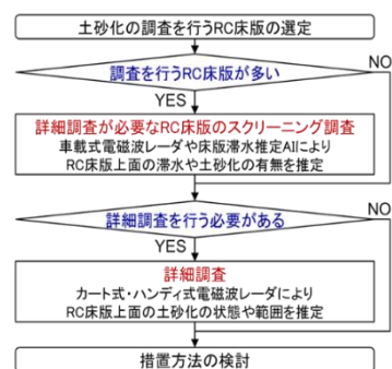
図-1 提案した土砂化の調査フロー
