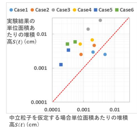
図-4 流木貯留高の水理実験結果と中立粒子仮定との比較
