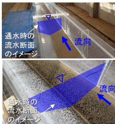
損傷実験前（上：通水前）後（下： 取水後）のモルタル水路（V字型）
